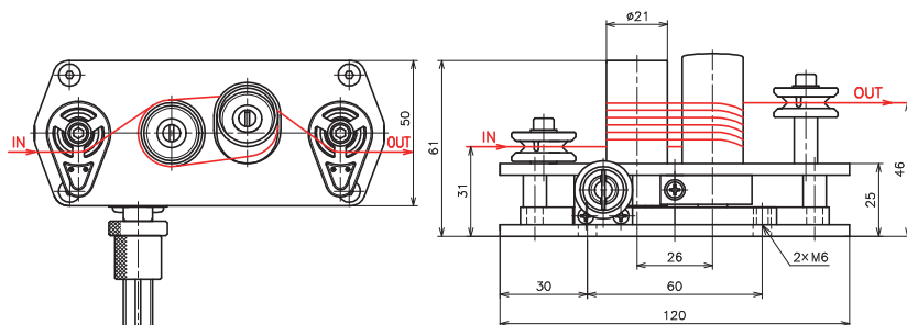
図面=D106020-R
