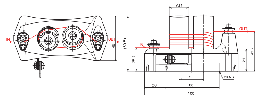
図面=D510060-R
